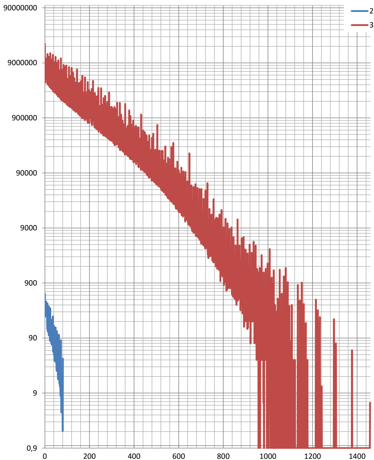
Рисунок 8.1. Зависимость логарифма количества матриц от модуля определителя по данным, представленным в таблицах 8.1 и 8.2
