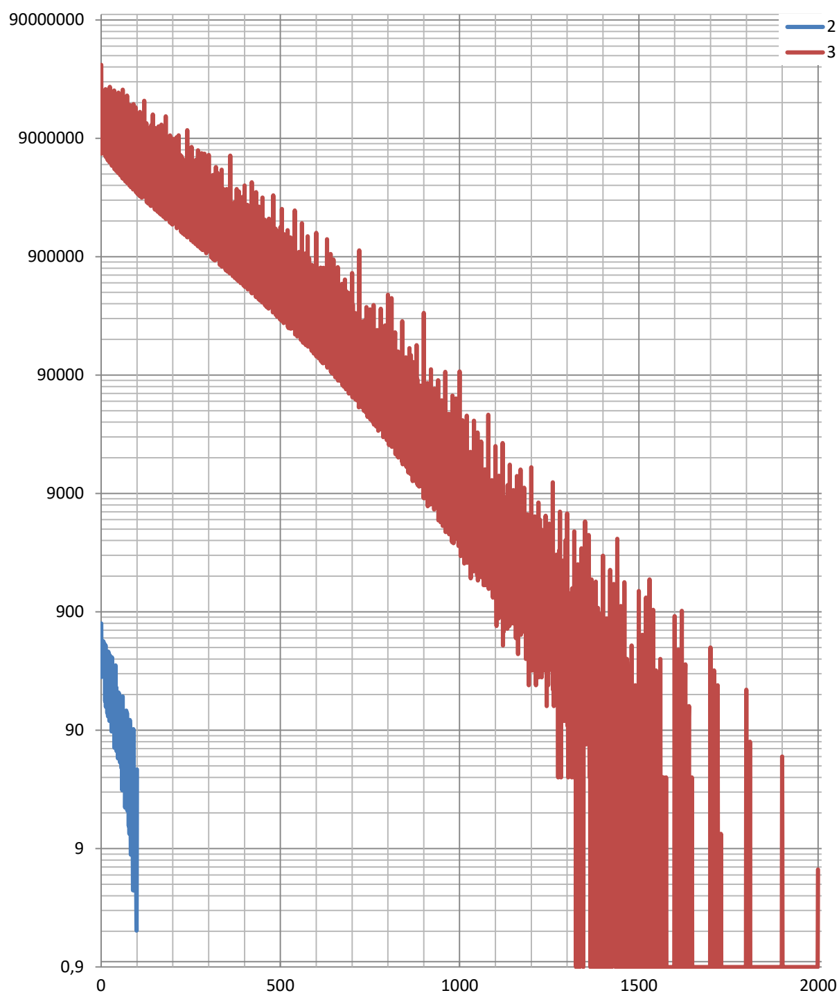
Рисунок 9.1. Зависимость логарифма количества матриц от модуля определителя по данным, представленным в таблицах 9.1 и 9.2
