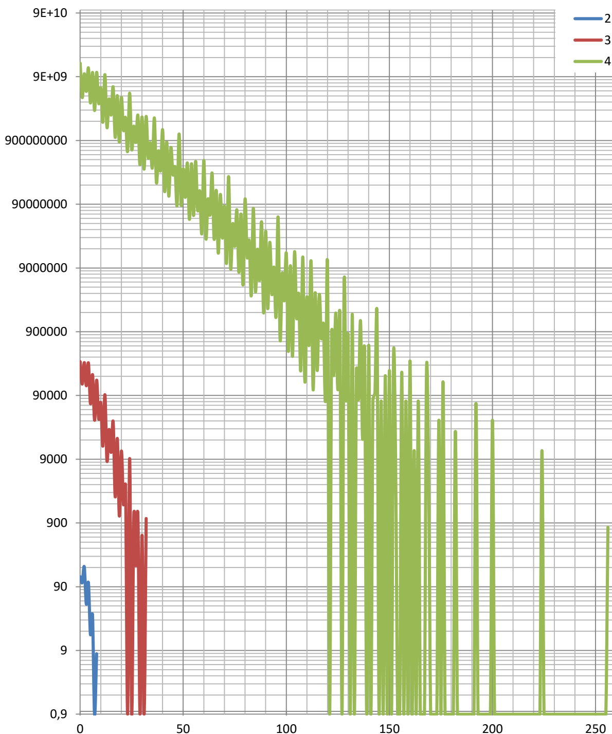
Рисунок 11.1. Зависимость логарифма количества матриц от модуля определителя по данным, представленным в таблицах 11.1–11.3
