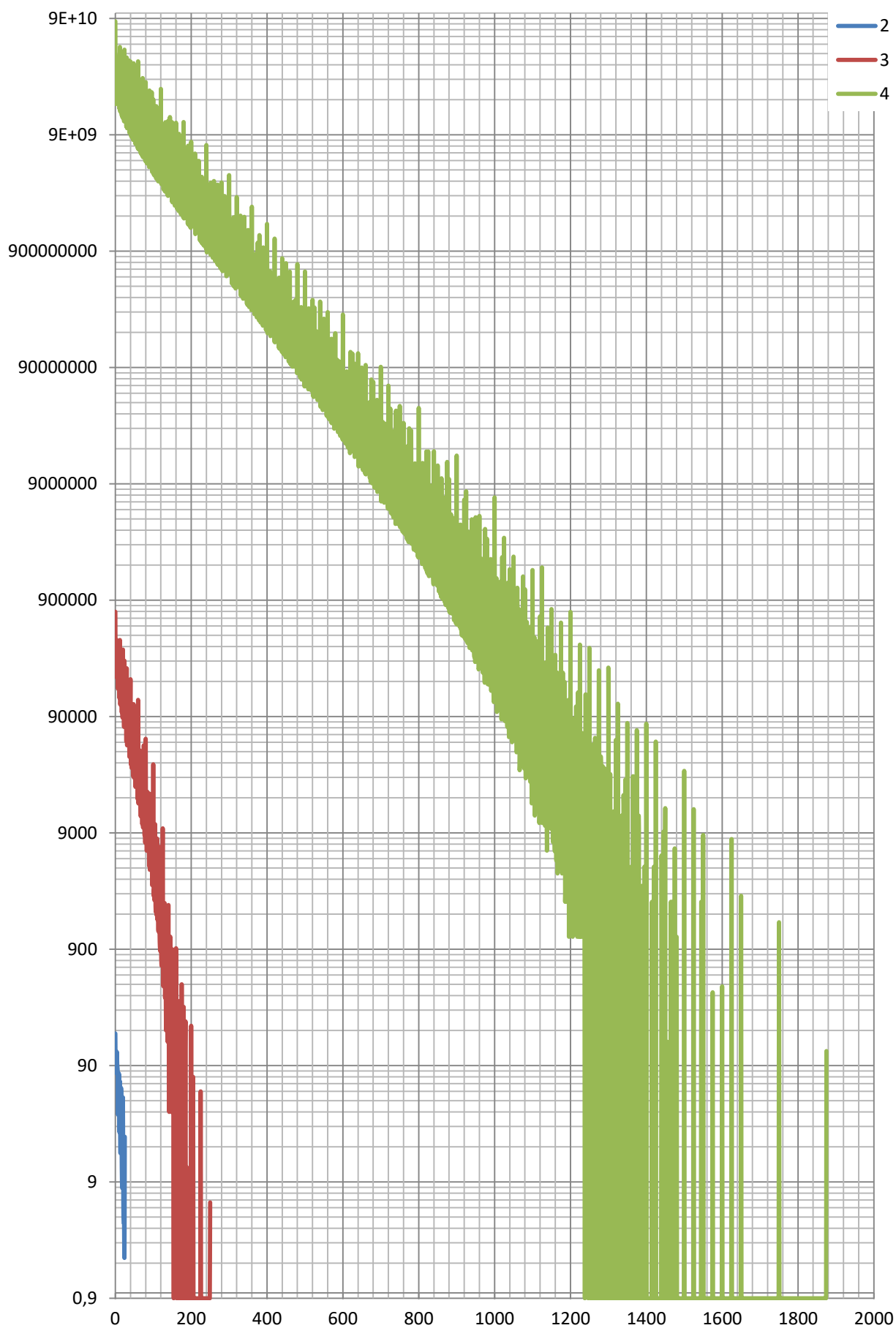
Рисунок 4.1. Зависимость логарифма количества матриц от модуля определителя по данным, представленным в таблицах 4.1–4.3
