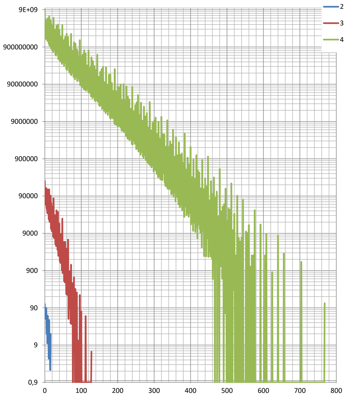
Рисунок 3.1. Зависимость логарифма количества матриц от модуля определителя по данным, представленным в таблицах 3.1–3.3
