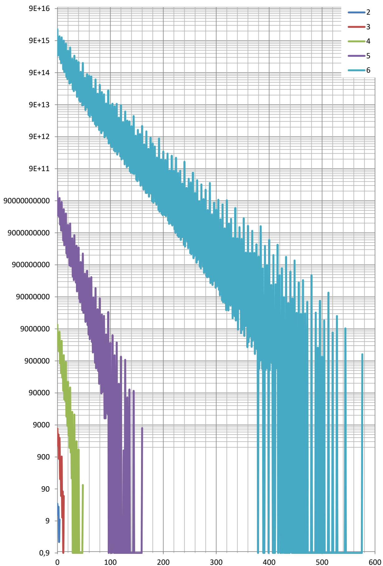
Рисунок 1.1. Зависимость логарифма количества матриц от модуля определителя по данным, представленным в таблицах 1.1–1.5
