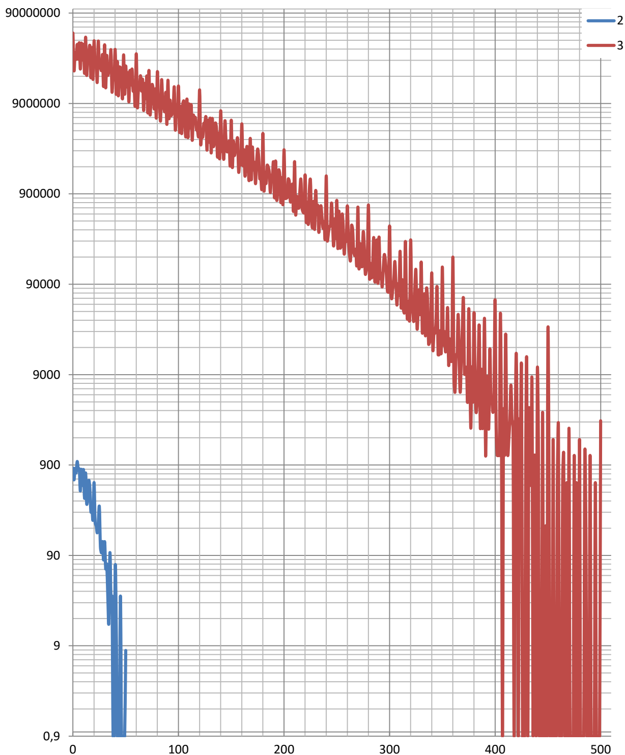
Рисунок 14.1. Зависимость логарифма количества матриц от модуля определителя по данным, представленным в таблицах 14.1 и 14.2
