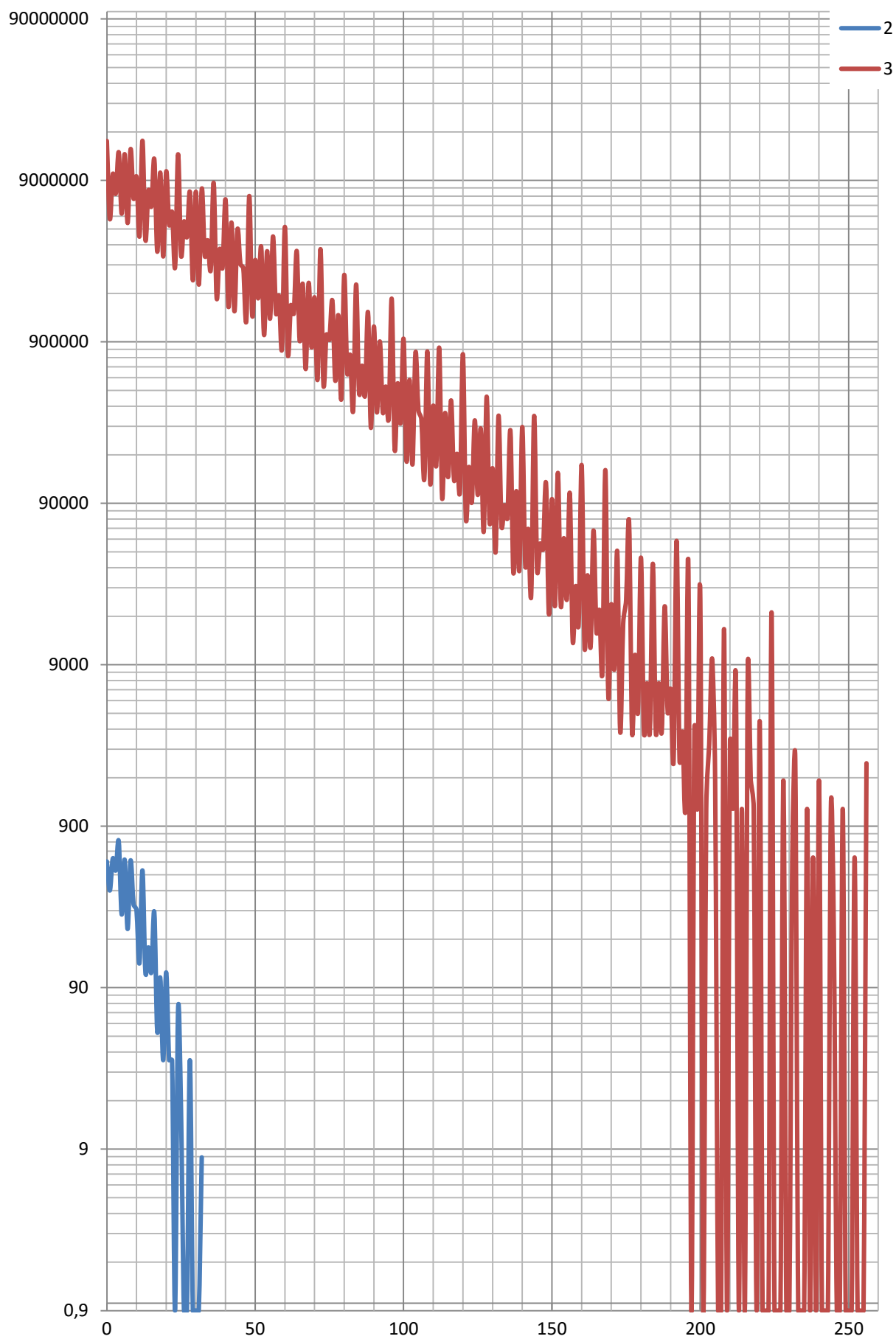
Рисунок 13.1. Зависимость логарифма количества матриц от модуля определителя по данным, представленным в таблицах 13.1 и 13.2
