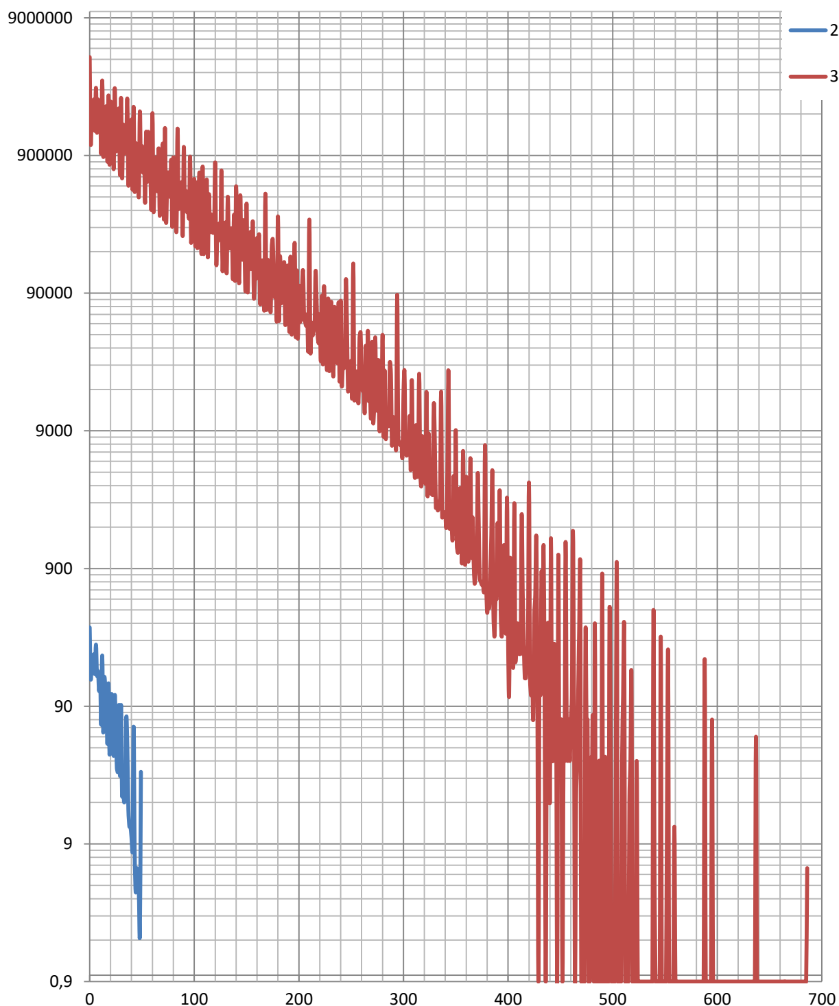
Рисунок 6.1. Зависимость логарифма количества матриц от модуля определителя по данным, представленным в таблицах 6.1 и 6.2
