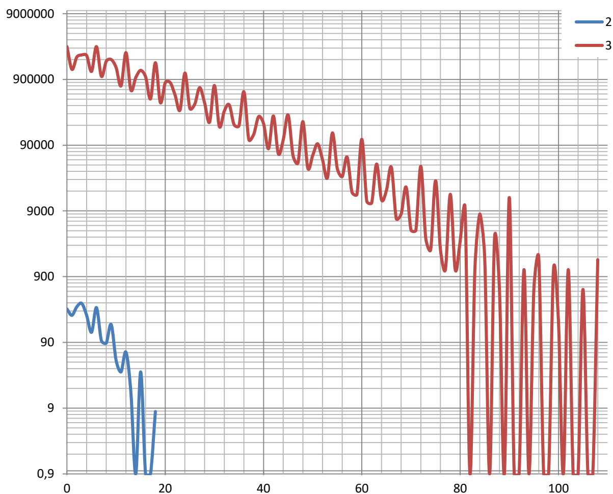
Рисунок 12.1. Зависимость логарифма количества матриц от модуля определителя по данным, представленным в таблицах 12.1 и 12.2
