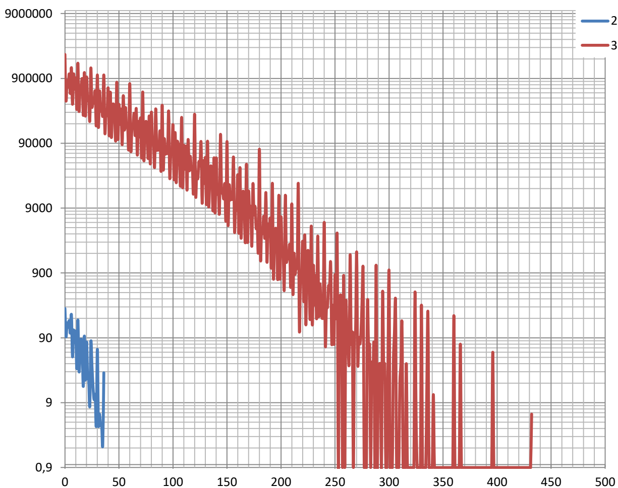
Рисунок 5.1. Зависимость логарифма количества матриц от модуля определителя по данным, представленным в таблицах 5.1 и 5.2
