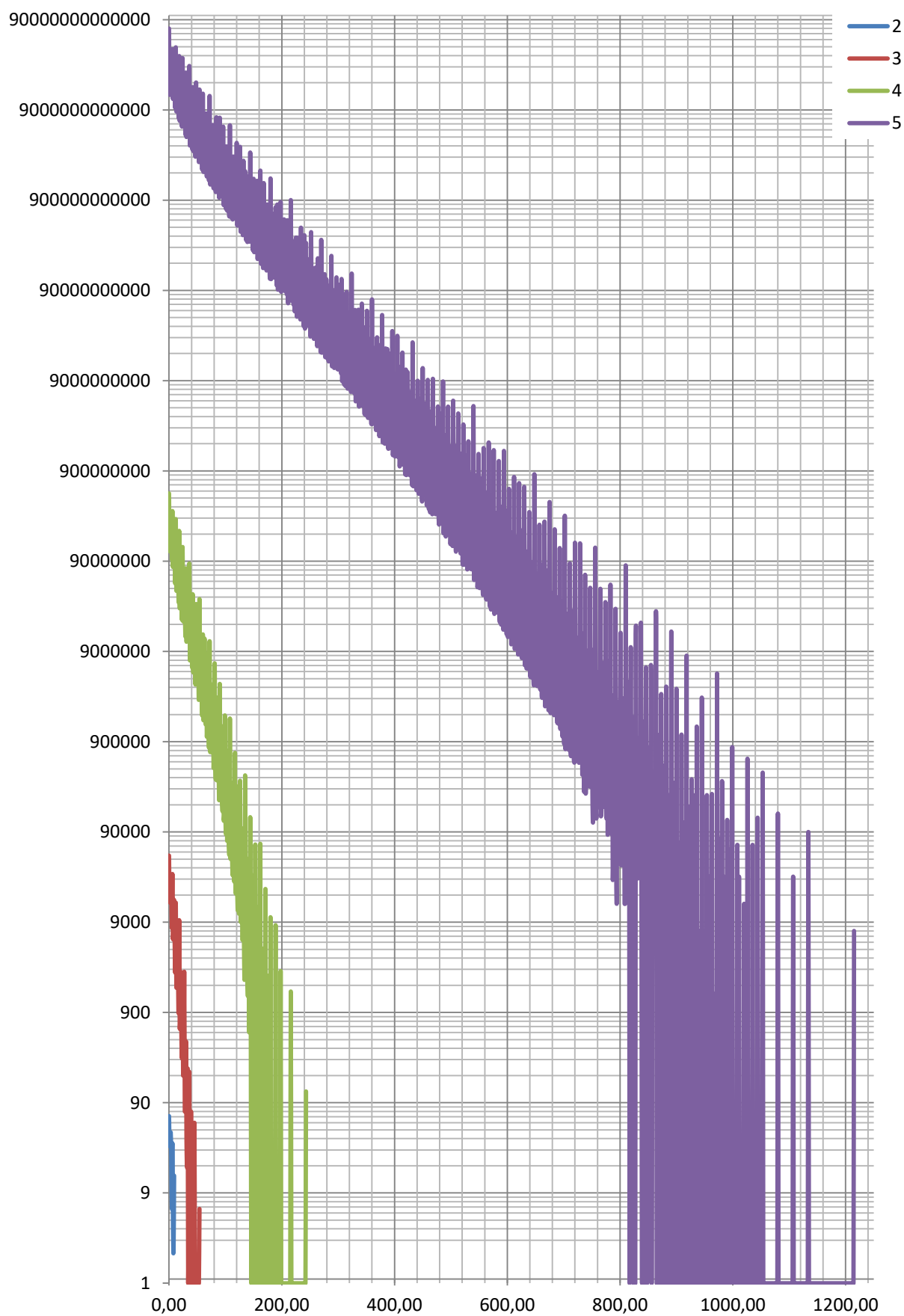
Рисунок 2.1. Зависимость логарифма количества матриц от модуля определителя по данным, представленным в таблицах 2.1–2.4
