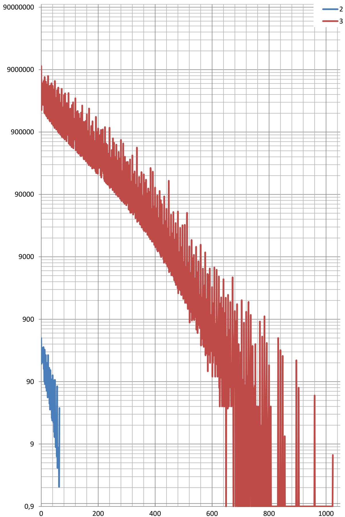
Рисунок 7.1. Зависимость логарифма количества матриц от модуля определителя по данным, представленным в таблицах 7.1 и 7.2
