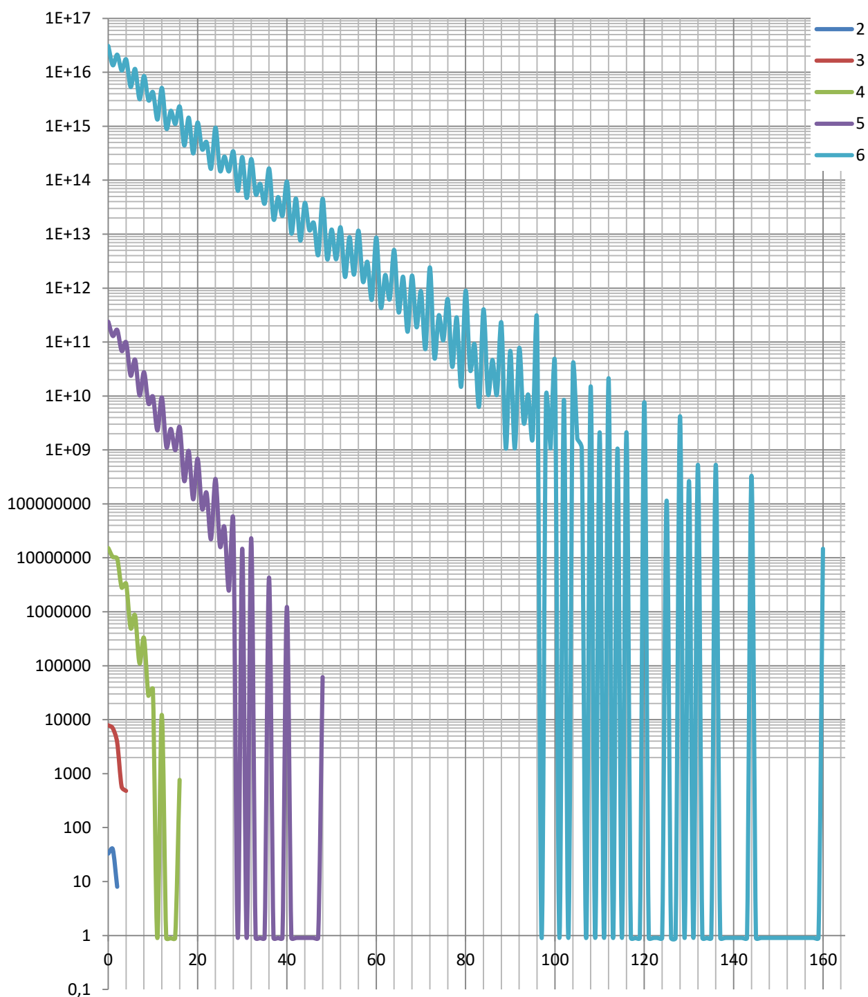
Рисунок 10.1. Зависимость логарифма количества матриц от модуля определителя по данным, представленным в таблицах 10.1–10.5
