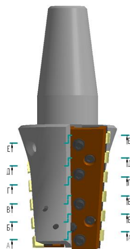
Рис. 2 – Разрезы секущих плоскостей фрезы
