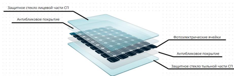
Рис. 1 – Схема оптимального размещения защитного антибликового покрытия «Sandwich» на монокристаллическую солнечную панель
