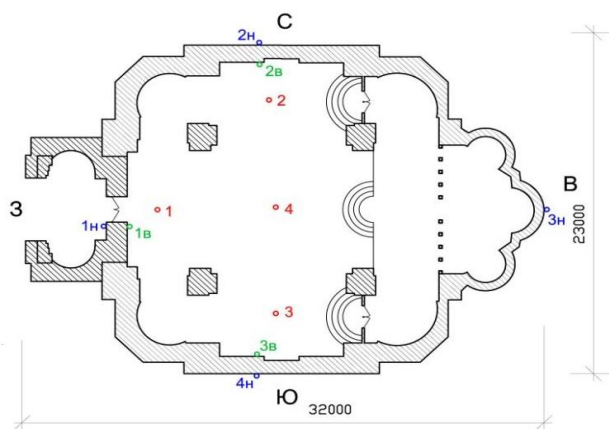
Рис. 1 – План Владимирского собора в г. Севастополе с маркировкой точек для массива данных
