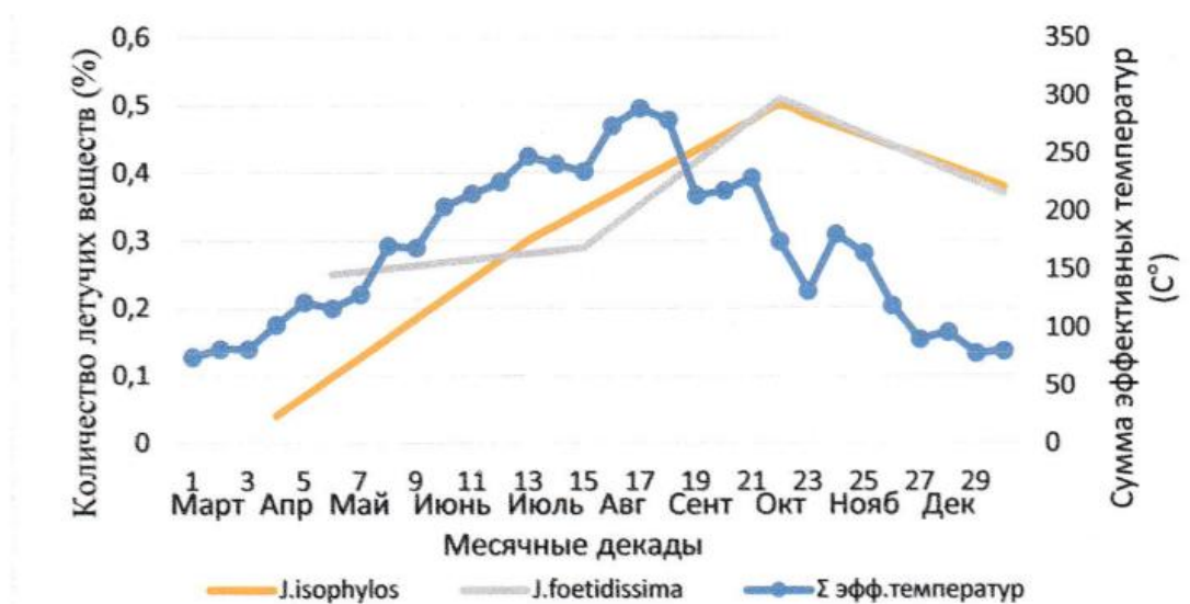
Рис. 1 – Зависимость выбросов БЛОС растениями рода Juniperus от расчетной СЭТ по декадам месяцев в 2023 году
